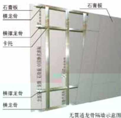
无贯通龙骨隔墙示意图
