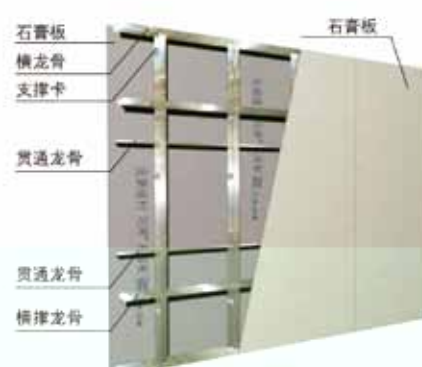
有贯通龙骨隔墙示意图
