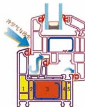
北新暖静门窗五腔室三密封结构图
